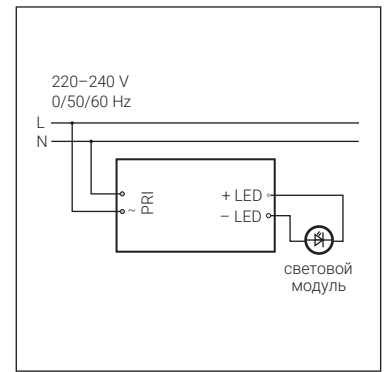
Схема подключения
